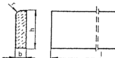
Rysunek 1. Kształt betonowego obrzeża chodnikowego
